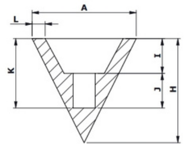
SECTION G-G SCALE 1 : 3
